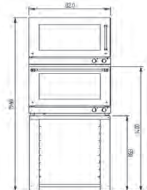
M 604 PLUS L M 604 PLUS STAND M 60_40 KIT SUPERPOSITION SERIES M 60_40
